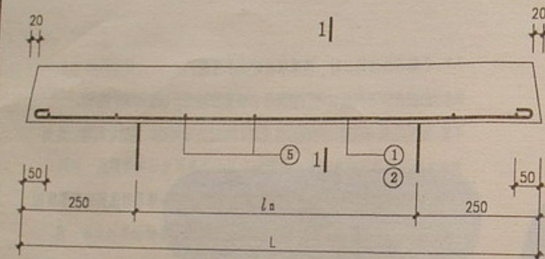
矩形板式过梁配筋大样A
