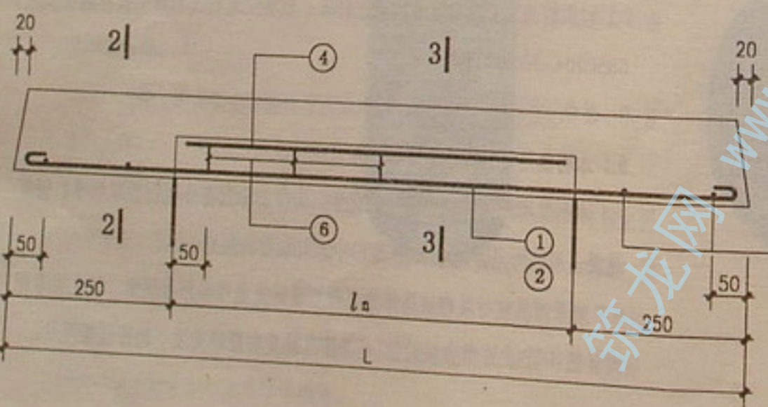
L形板式过梁配筋大样B
